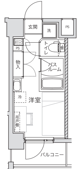
C2type 居室面積 13.19m 2
