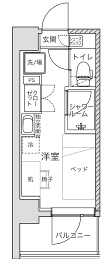
Atype 居室面積 13.29㎡
