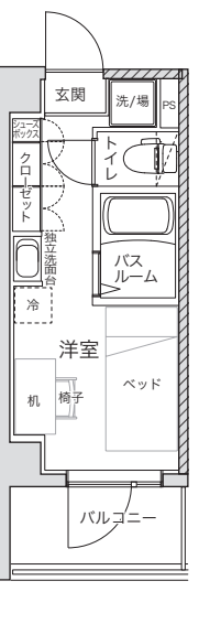
Ptype 居室面積 13.47㎡
