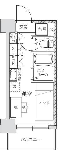
Ltype 居室面積 13.35㎡
