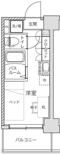
Ctype 居室面積 13.29㎡
