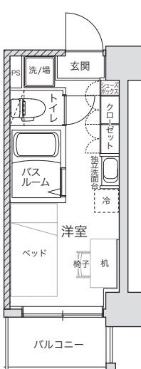
Itype 居室面積 13.35㎡
