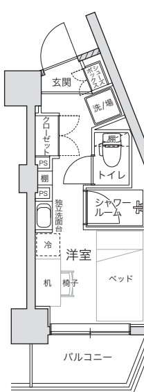
Ntype 居室面積 13.93㎡
