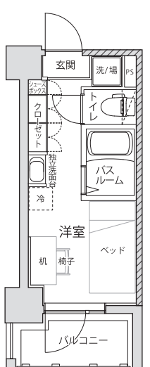
J type 居室面積 13.35㎡
