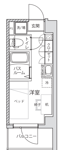
O type 居室面積 13.43㎡
