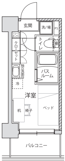
D type 居室面積 13.35㎡
