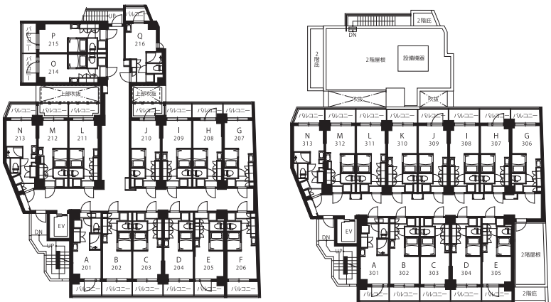
2F
