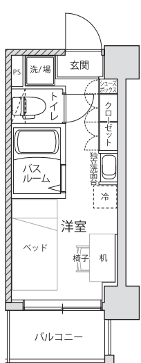
I type 居室面積 13.35㎡
