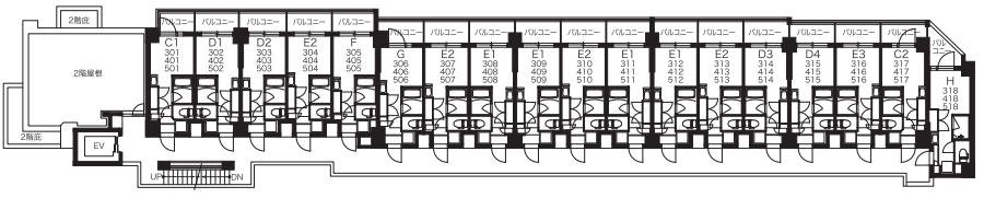
3F~5F
