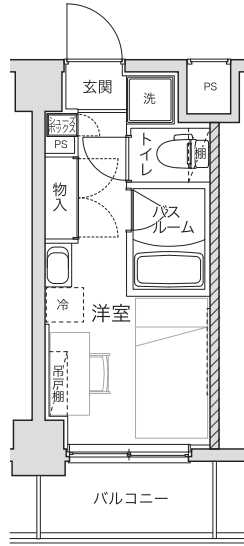
D1type 居室 12.90㎡
