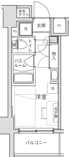
Ftype 居室 12.91㎡
