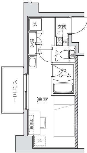
Atype 居室 15.60㎡
