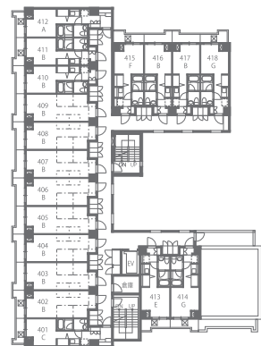
[4F 平面図]
