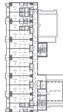
[6F 平面図]
