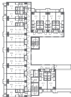
[4F 平面図]
